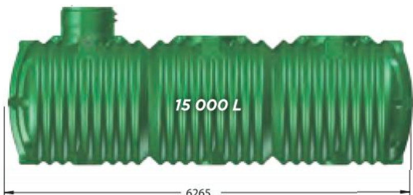
ET15000, poids : 649 kg
