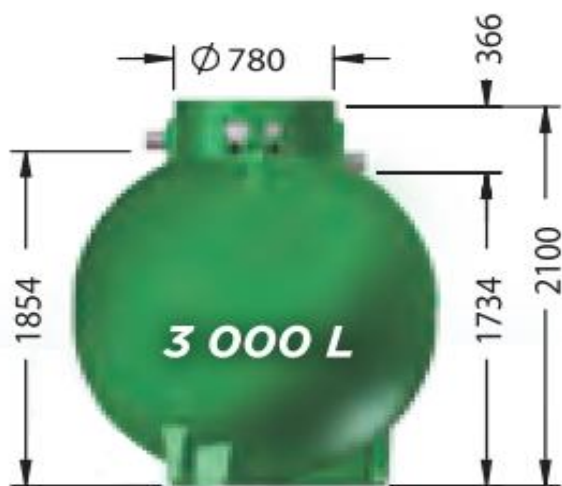
ET03000, poids : 116 kg
