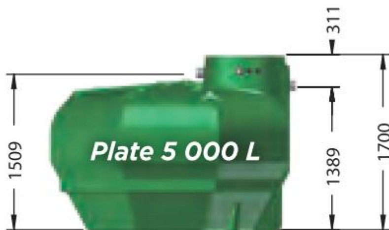
ETS05000 , poids : 220 kg
