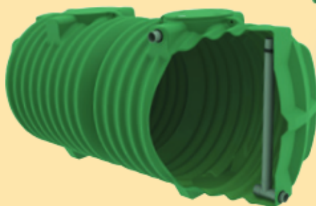
Détail de l'ajutage réglable
